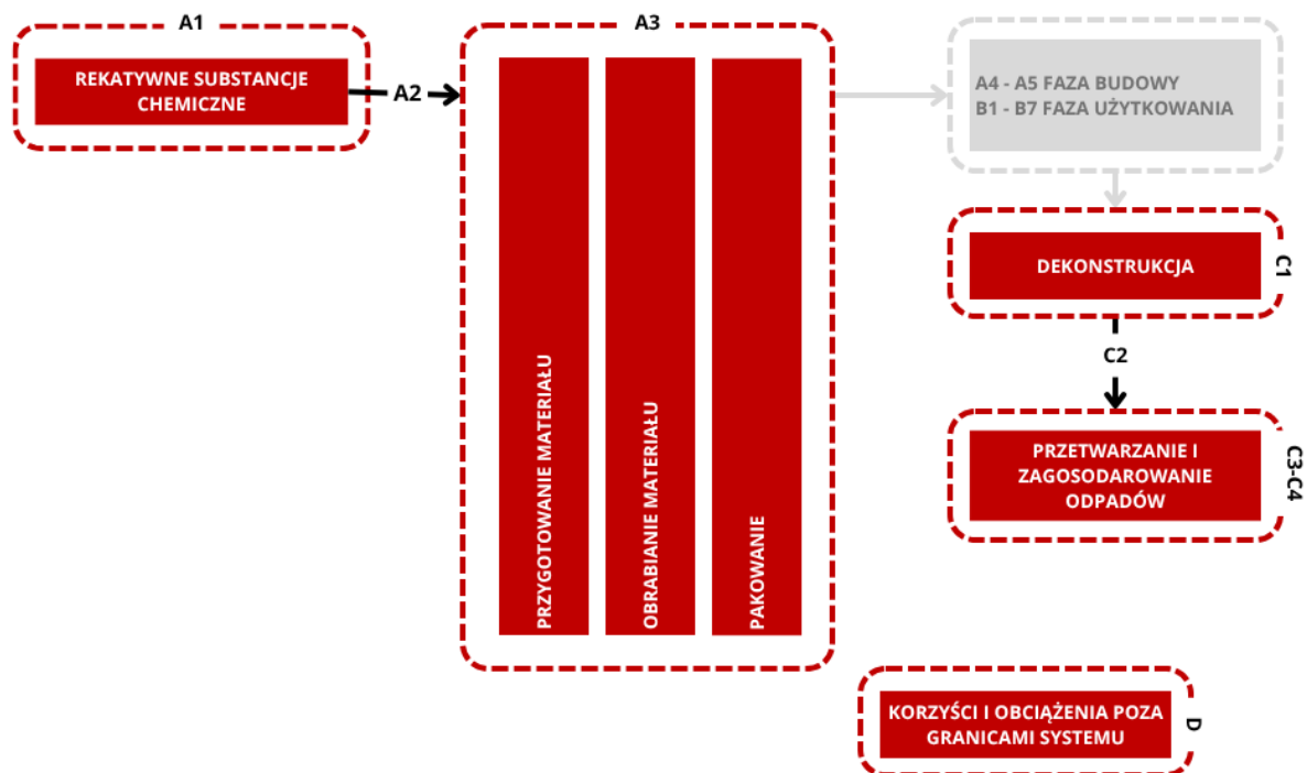
Rysunek 5.1: Granice systemu dla charakterystyki środowiskowej dysków pęczniejących
